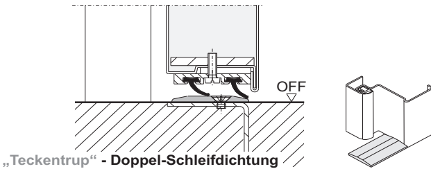
„Teckentrup“ - Doppel-Schleifdichtung Zarge mit Bodeneinstand zwingend erforderlich
