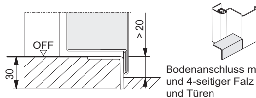
absenkbare Bodendichtung
