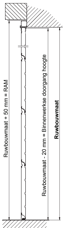
Inbouw achter de dag, alleen naar binnen openend
